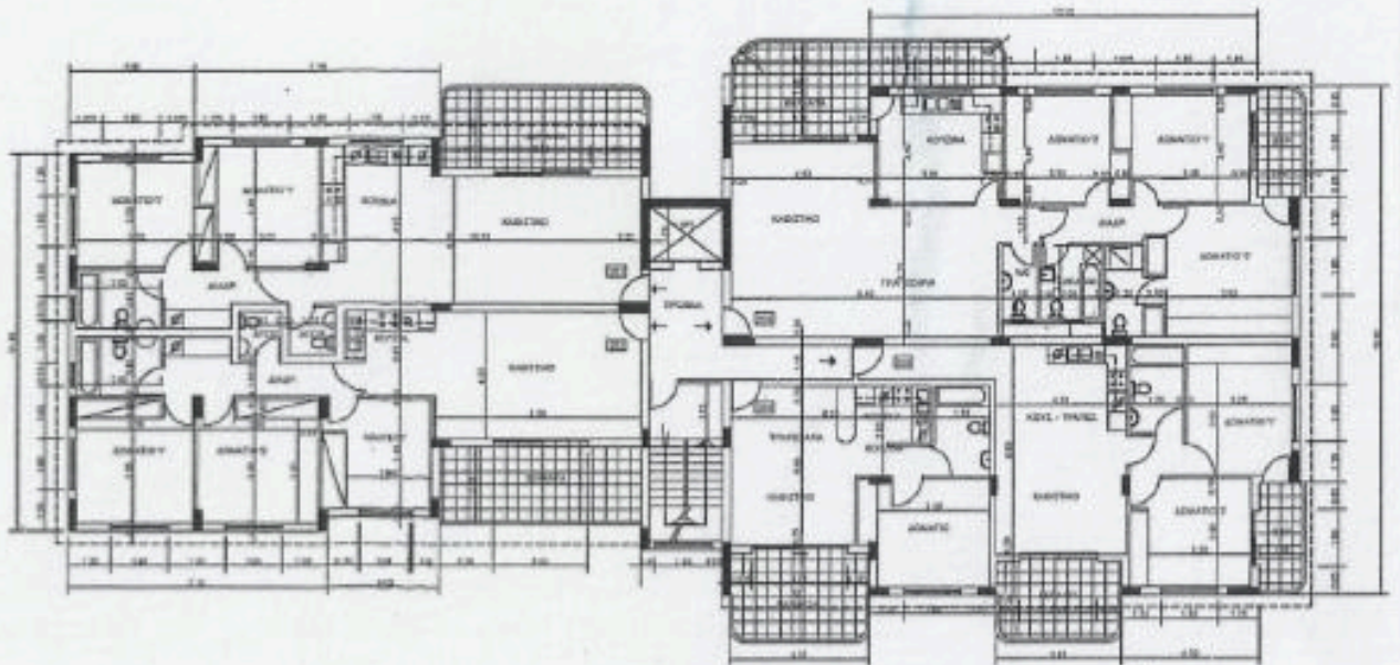
ΚΑΤΩΦΗ Ε. ΟΡΟΦΟΥ ΚΑΙΝΑΚΑ 1:100
