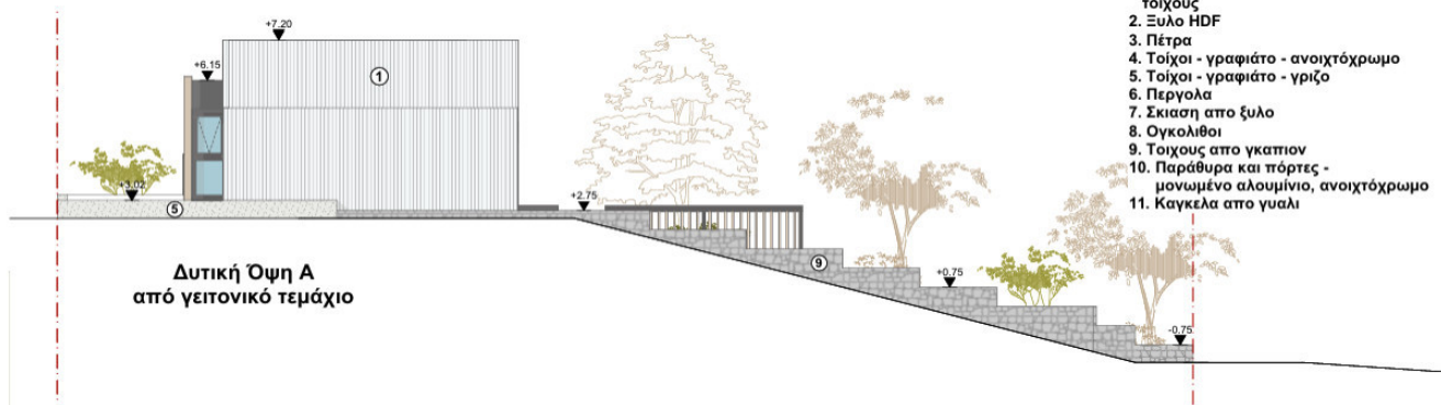
Δυτική Όψη
